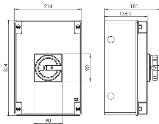
Abmessungen Gehäuse PM-D3 Dimensions enclosure PM-D3
